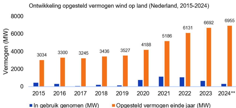
Figuur 5.4: Jaarlijks opgesteld vermogen en netto toename wind op land. (CBS, 2025c).
